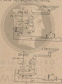
Σχῆμα 3. — Χειριστήριον.
