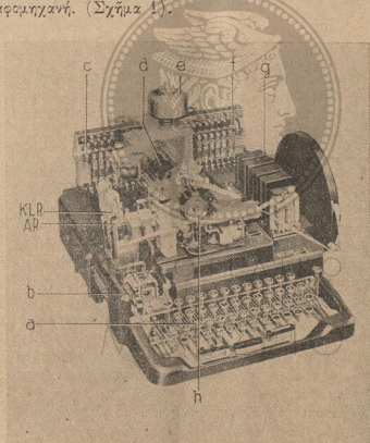
Σχῆμα 1. = Τηλεγραφομηχανή.
